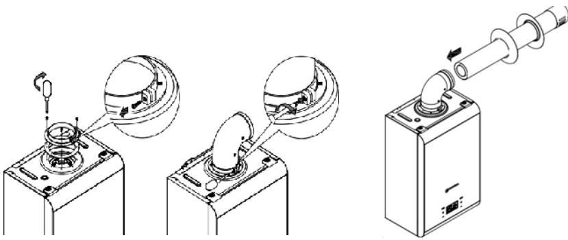
Figura 28: Instalación del conjunto de piezas
