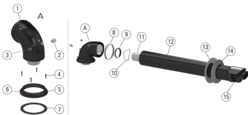
Figura 27: chimenea
