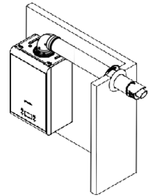
Figura 29: Salida concéntrica de la chimenea
