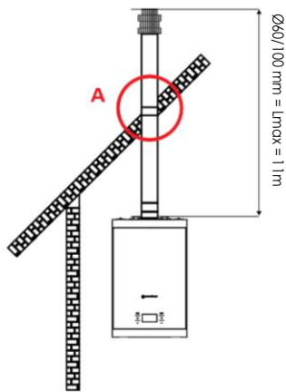
Figura 35: Instalación de chimenea vertical
