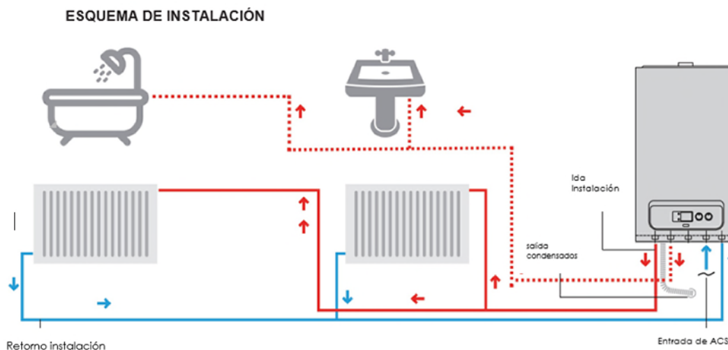
Figura 17: Esquema de instalación
