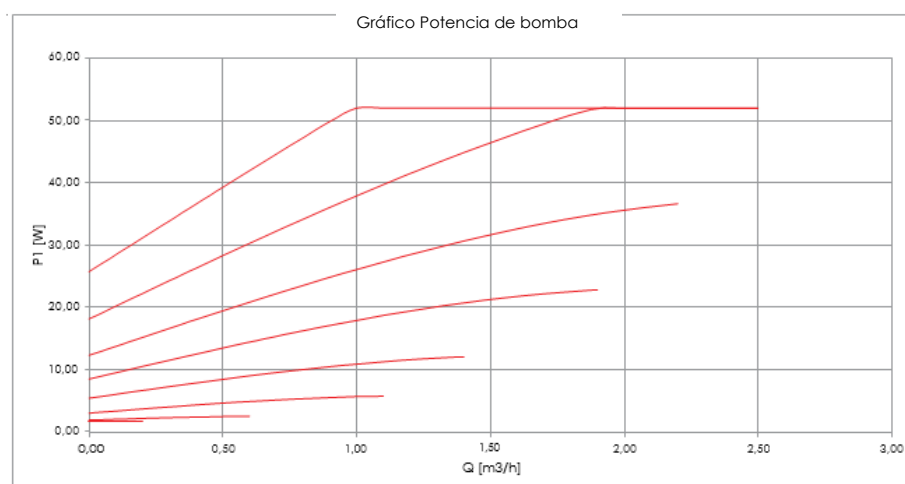
Figura 8: Gráficos de altura y potencia de bomba MINERWA
