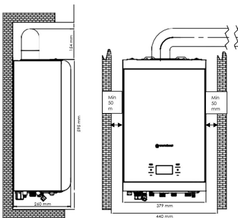
Figura 10: Dimensiones mínimas del alojamiento
