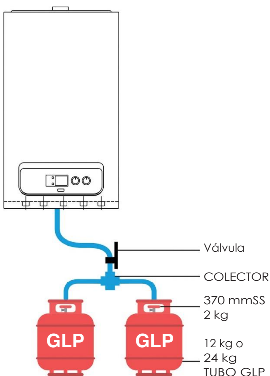
Figura 12: Conexión de la caldera a botellas de gas
