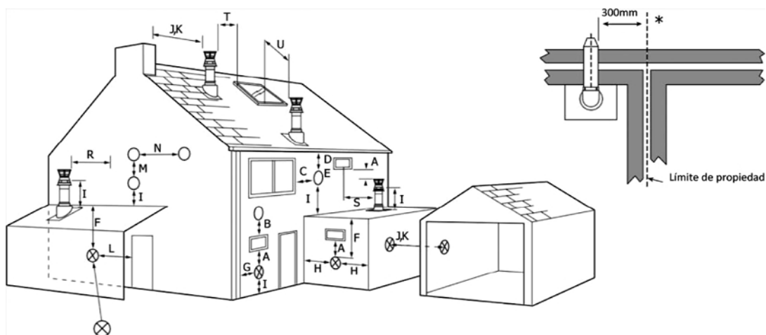
Figura 26: Posiciones periféricas de la chimenea
