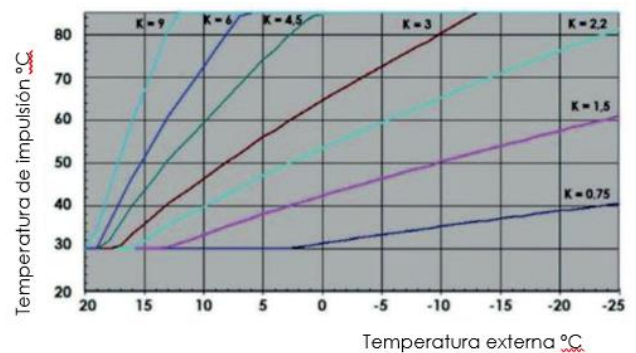
Figura 44: Curvas de operación de la sonda externa
