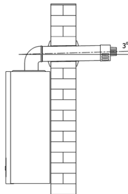
Figura 30: Inclinación de la chimenea de condensación de la caldera
