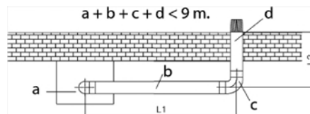
Figura 33: Instalación de chimenea coaxial con dos codos de 90°
