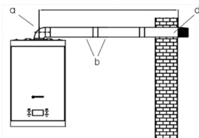
Figura 32: Instalación de chimenea simple con codo de 90°
