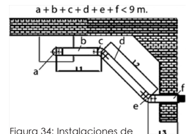
Figura 34: Instalaciones de chimenea coaxial con un codo de 90° y dos codos de 45°
