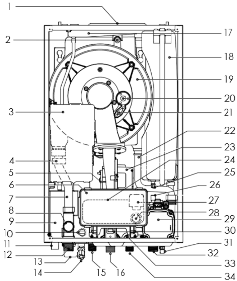
Figura 6: Componentes de caldera
