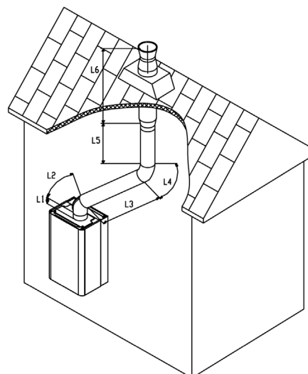
Figura 37: Aplicación de chimenea vertical
