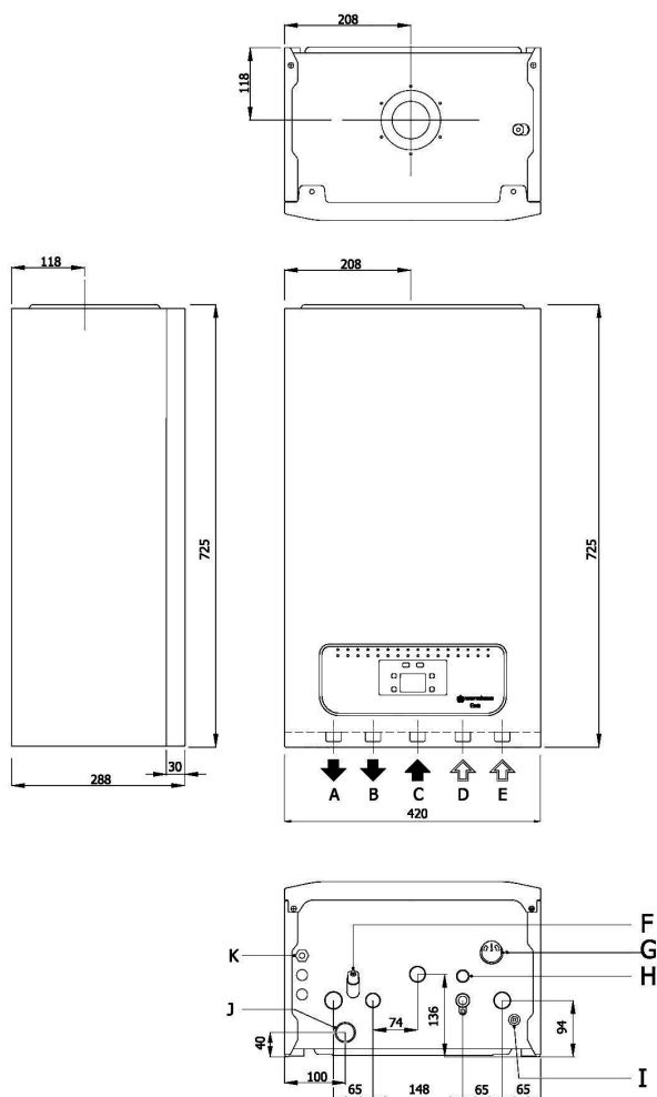
Figura 11: Dimensiones y conexiones EWA
