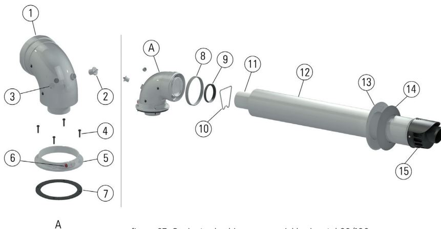
figura 27: Conjunto de chimenea coaxial horizontal 60/100
