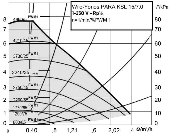
Figura 8: Gráfico de Presión/Caudal de bomba EWA
